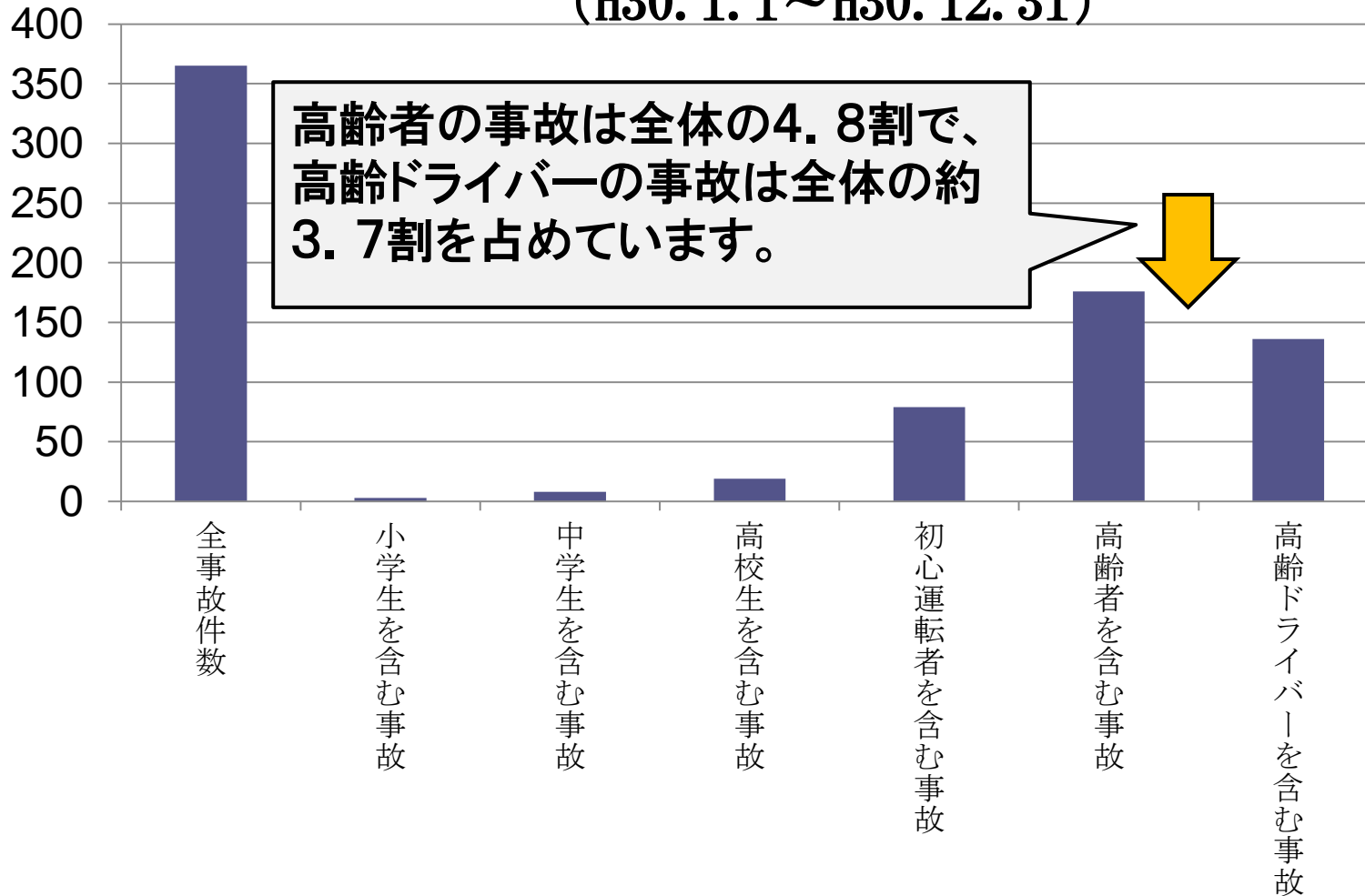
新居浜警察署管内交通事故発生件数（年齢別） （H30. 1. 1～H30. 12. 31）
